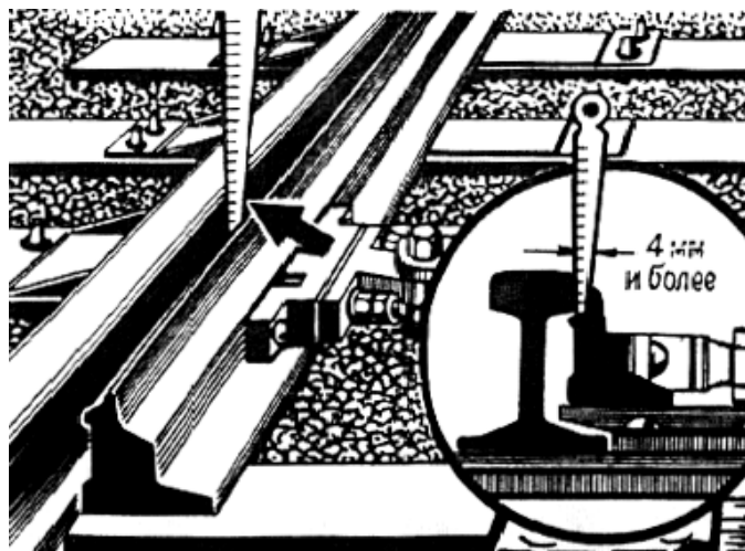
Рисунок 3 – Отставание остряка от рамного рельса
