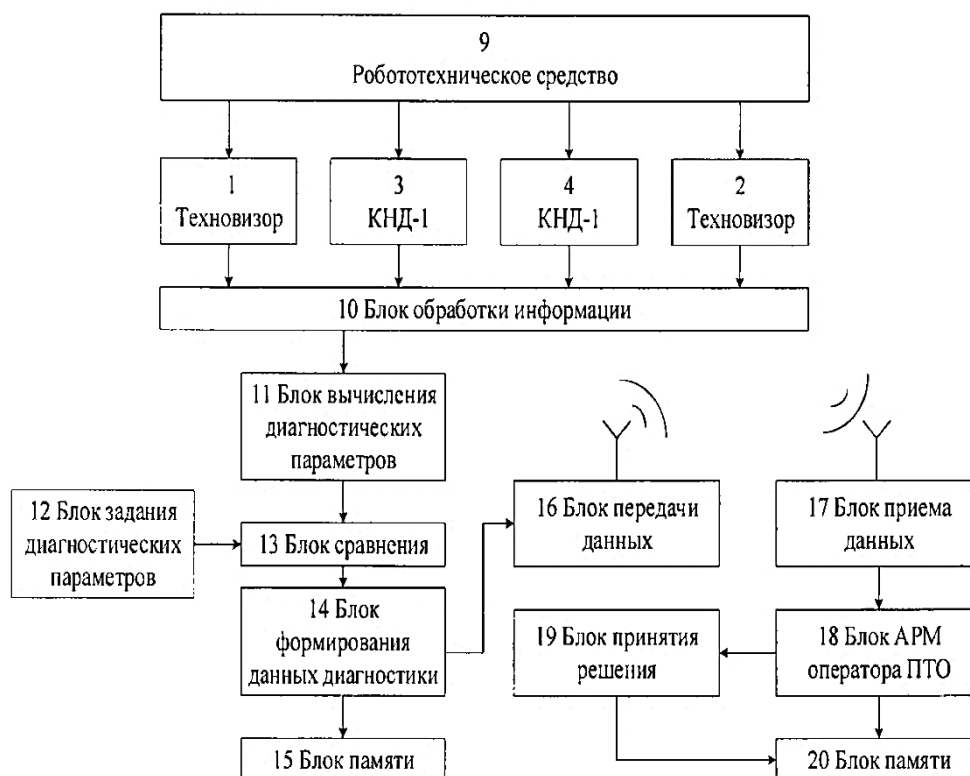
Рисунок 3 – Схема работы роботизированного контроля технического состояния вагонов
