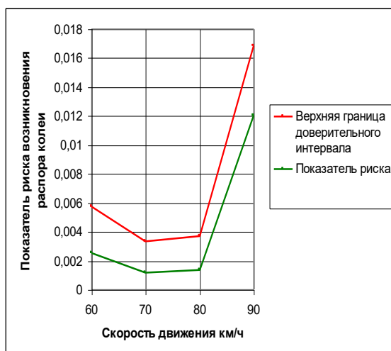
Зависимость показателя риска возникновения распора колеи от скорости движения
