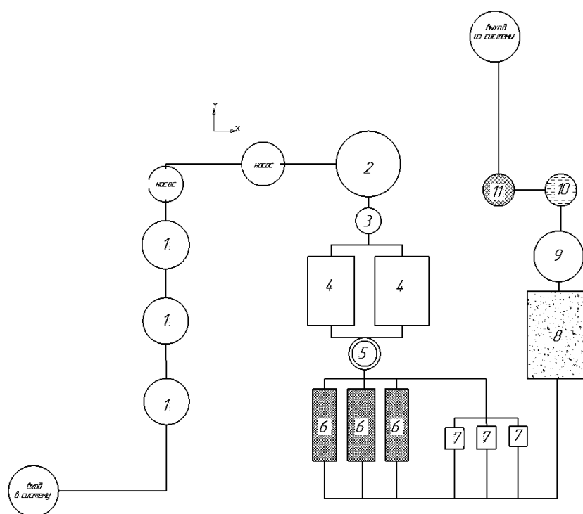
Рисунок 1 – Принципиальная технологическая схема последовательности работы очистных сооружений: 1 – малый накопительный резервуар; 2 – большой накопительный резервуар; 3 – приёмная камера; 4 – нефтеуловитель; 5 – канализационная насосная станция; 6 – флотатор ФФУ-20; 7 – фильтр ФСД-20; 8 – биореактор; 9 – колодец сброса чистой воды; 10 – колодец коллектора НГЧ-7, 11 – колодец подачи стоков на мойку тепловозов для повторного использования
